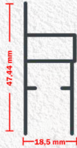
Ürün (SKU): 124 Ağırlık (Weight): 267 gr / m. 18 MM PLİSE SİNEKLİK İÇTEN TAKMA KASA PROFİLİ SLIM PLEATED FS INSIDE MOUNTED FRAME PROFILE
