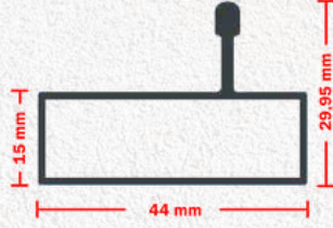
Ürün (SKU): 151 Ağırlık (Weight): 400 gr / m. SÜRME TEKLİ RAY PROFİLİ SINGLE RAIL PROFILE FOR SLIDING FLY SCREEN
