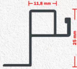
Ürün (SKU): 131 Ağırlık (Weight): 250 gr / m. İÇTEN TAKMA SİNEKLİK PROFİLİ PRACTICAL FLY SCREEN PROFILE (INSIDE MOUNTED)
