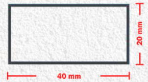
Ürün (SKU): 171 Ağırlık (Weight): 292 gr / m. 20X40 KUTU PROFİLİ 20X40 FRAME PROFILE
