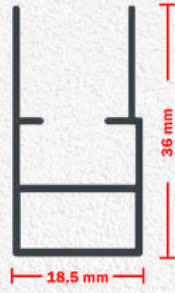
Ürün (SKU): 121 Ağırlık (Weight): 258 gr / m. 18 MM PLİSE SİNEKLİK KASA PROFİLİ SLIM PLEATED FLY SCREEN FRAME PROFILE
