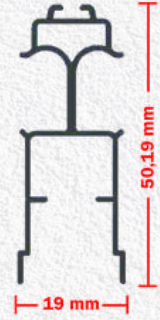
Ürün (SKU): 122 Ağırlık (Weight): 358 gr / m. 18 MM PLİSE SİNEKLİK KANAT PROFİLİ SLIM PLEATED FLY SCREEN SLIDING PROFILE
