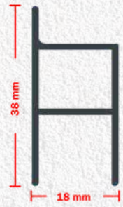
Ürün (SKU): 127 Ağırlık (Weight): 265 gr / m. M2 PLİSE SİNEKLİK İÇTEN TAKMA KASA PROFİLİ M2 SLIM PLEATED FS INSIDE MOUNTED FRAME PROFILE
