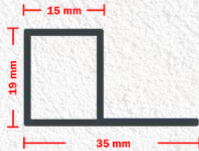
Ürün (SKU): 143 Ağırlık (Weight): 234 gr / m. İÇE AÇILIM P PROFİLİ P PROFILE FOR HINGED FS OPENS INSIDE
