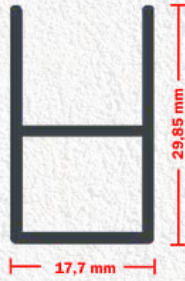
Ürün (SKU): 125 Ağırlık (Weight): 217 gr / m. M2 18 MM PLİSE SİNEKLİK KASA PROFİLİ M2 SLIM PLEATED FLY SCREEN FRAME PROFILE
