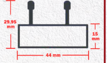
Ürün (SKU): 152 Ağırlık (Weight): 550 gr / m. SÜRME ÇİFTLİ RAY PROFİLİ DOUBLE RAIL PROFILE FOR SLIDING FLY SCREEN
