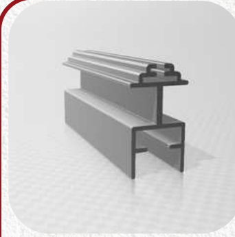
Ürün (SKU): 126 Ağırlık (Weight): 284 gr / m. M2 18 MM PLİSE SİNEKLİK KANAT PROFİLİ M2 SLIM PLEATED FLY SCREEN SLIDING PROFILE
